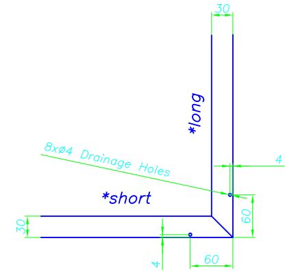
DETAIL A (x4 SCALE)
